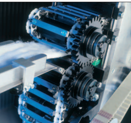
Watteband-Einzug
