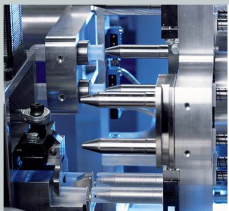
Montage-Einheit
