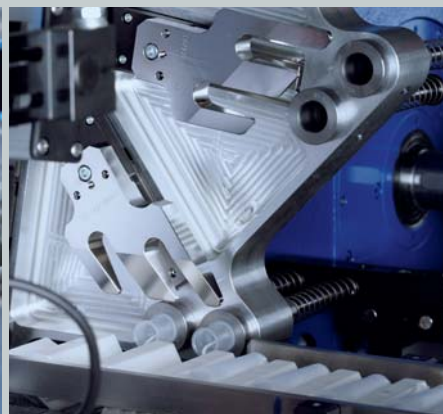
Transport-Trommel
