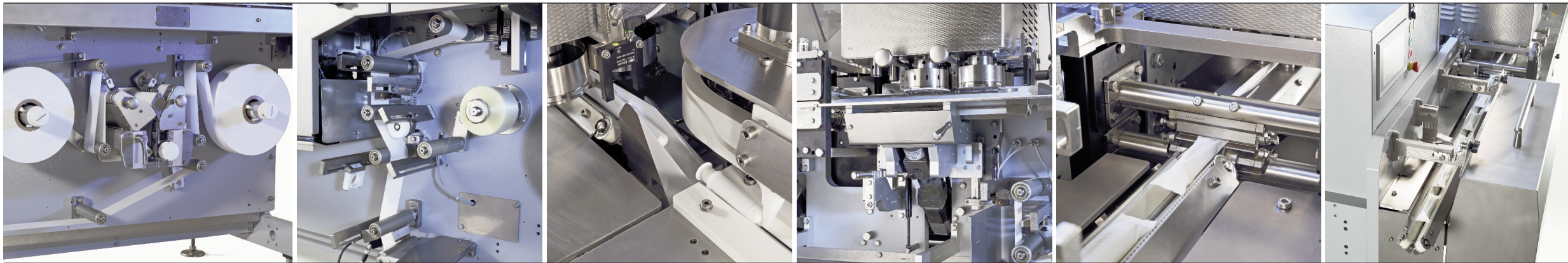
Splicing unit Spleiss-Einheit Web guide control Bahnlaufsteuerung Folding box Faltkasten Length sealing unit Längssiegel-Einheit Cross sealing unit Quersiegel-Einheit Output conveyor Auslaufband
